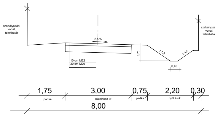
mezőgazdasági út tervezett kiszolgáló út mintakeresztmetszéje egyoldali árokkal K.VIII.
