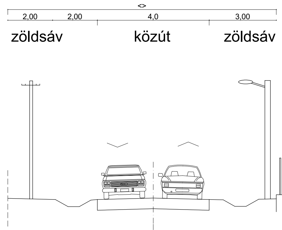
Tervezett 87106 j. bek. út mintakeresztmetszéje belterületen
